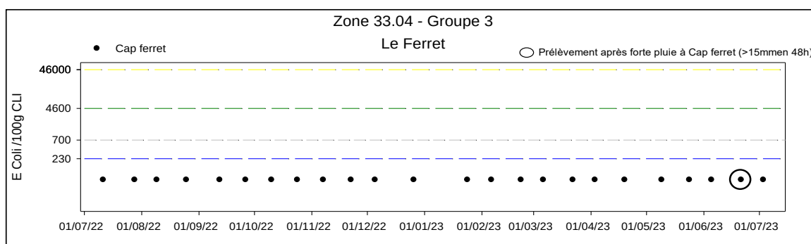
Figure 51 : Résultats des analyses en E. coli au point 087-P-001 « Cap Ferret (a) ».
