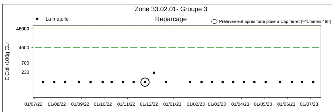
Figure 49 : Résultats des analyses en E. coli au point 088-P-166 « La Matelle ».
