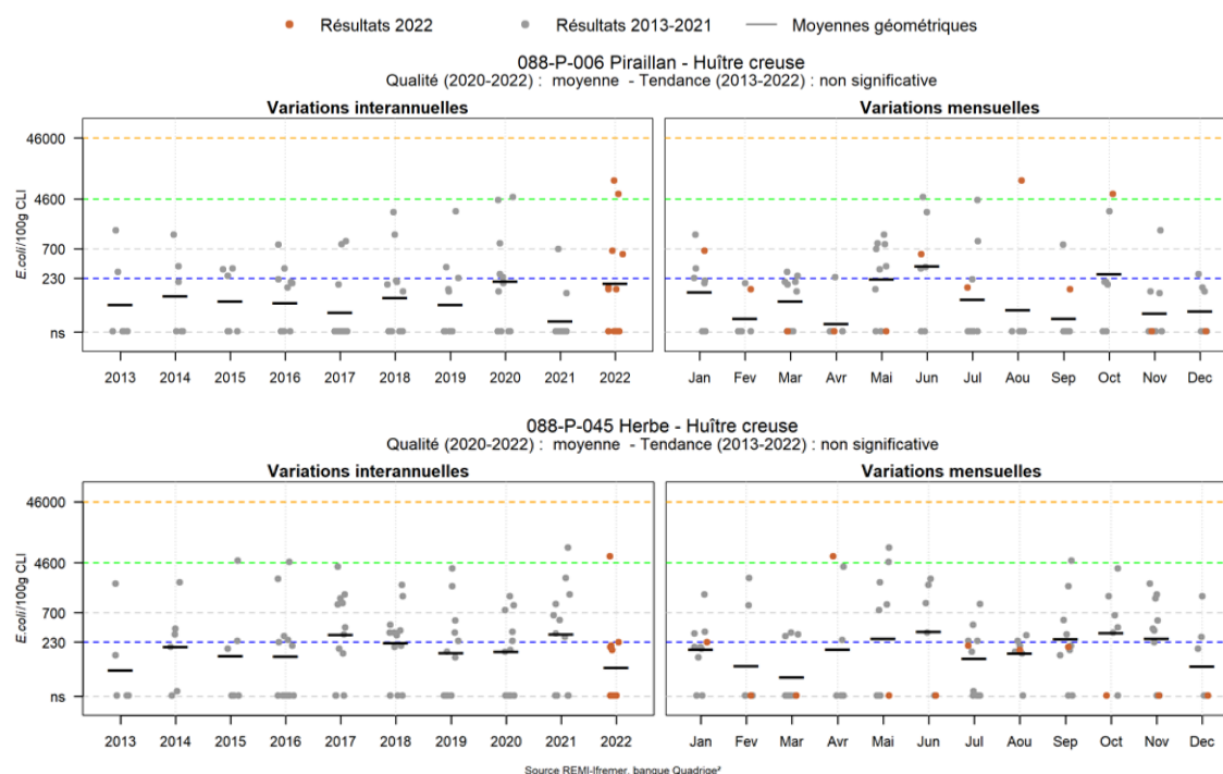
Figure 34 : Résultats REMI des huîtres – Zone 33.05 - Pirailan (source : Ifremer)
