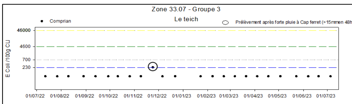
Figure 53 : Résultats des analyses en E. coli au point 088-P-021 « Comprian(a) ».
