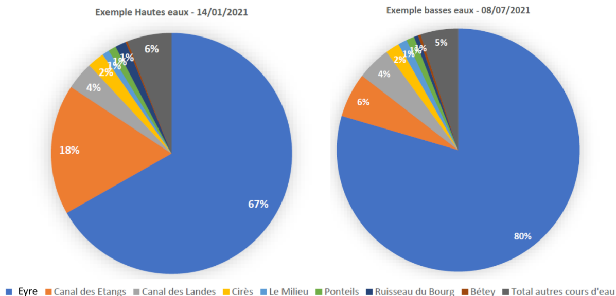
Figure 43 : Représentation graphique des débits des principaux cours d'eau du Bassin d'Arcachon (source : SIBA-REMPAR)
