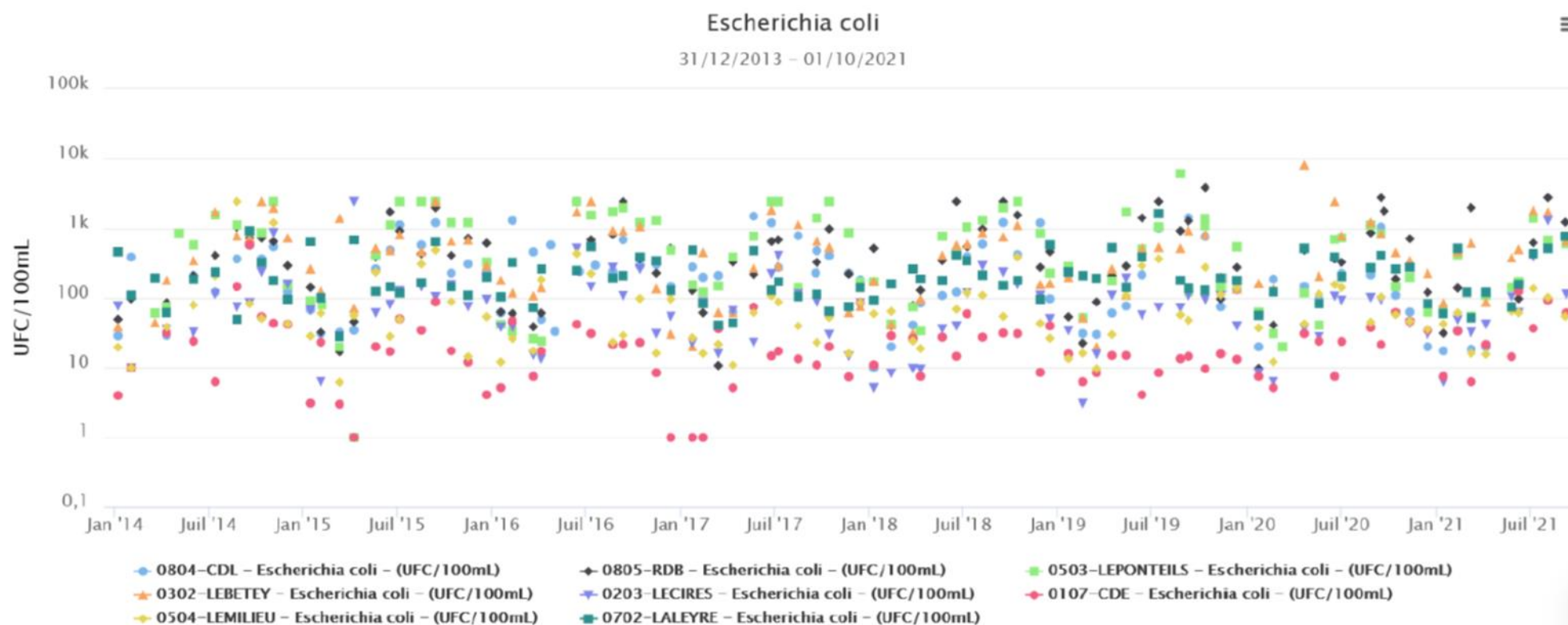
Figure 41 : Concentration E. coli des principaux tributaires du Bassin d'Arcachon de 2014 à 2021 en échelle logarithmique (source : SIBA-REMPAR)
