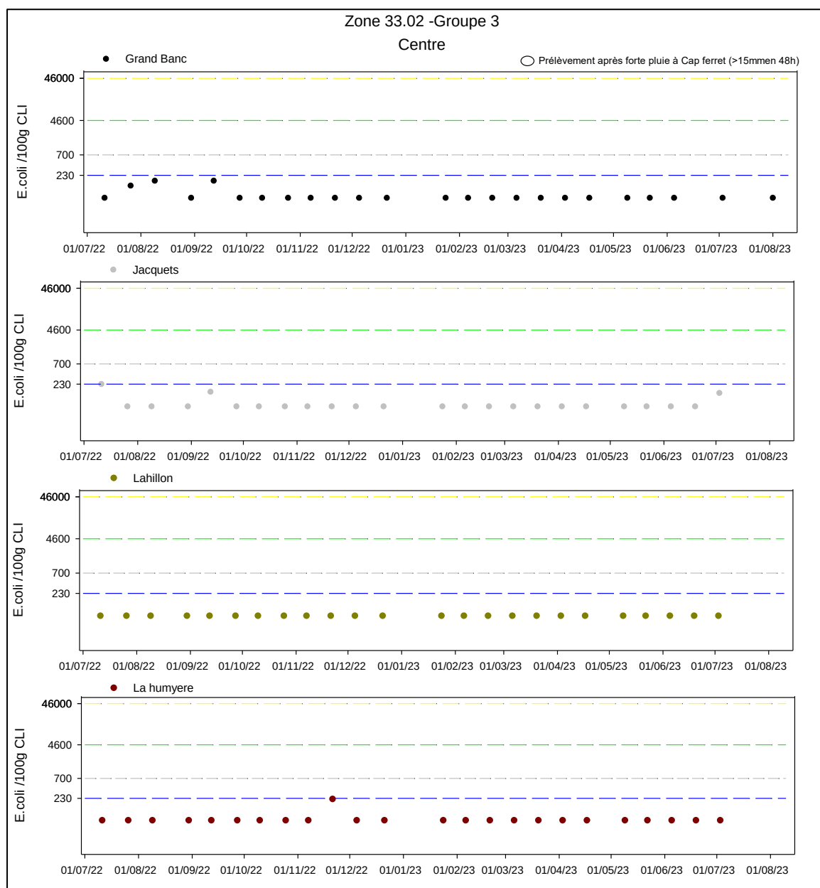
Figure 48 : Résultats des analyses en E. coli aux points « 088-P-035 Grand Banc », « 088-P-007 Jacquets aval », « 088-P-164 La Humeyre » et 088-P-165 « Lahillon (a) ».
