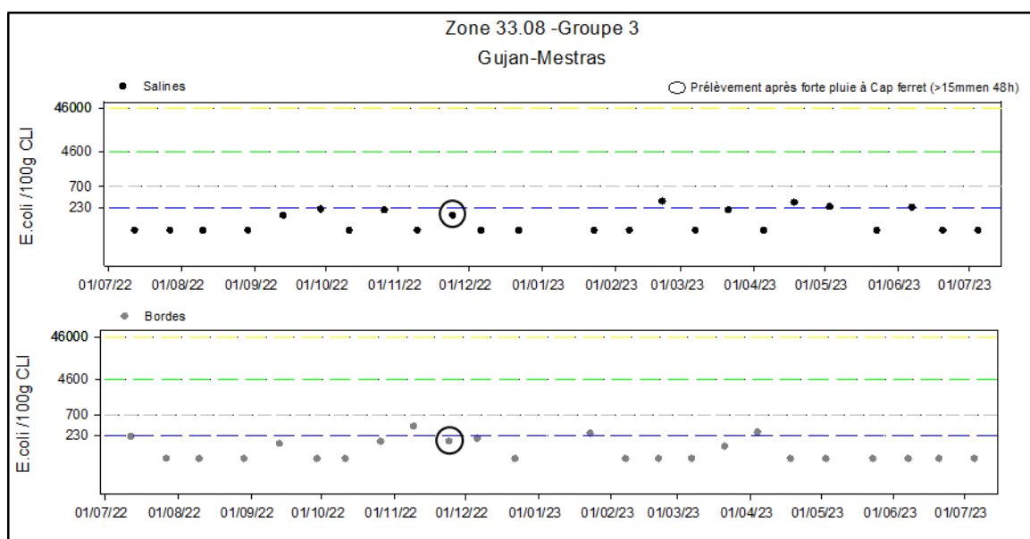
Figure 54 : Résultats des analyses en E. coli aux points « 088-P-161 Salines » et « 088-P-026 Bordes ».
