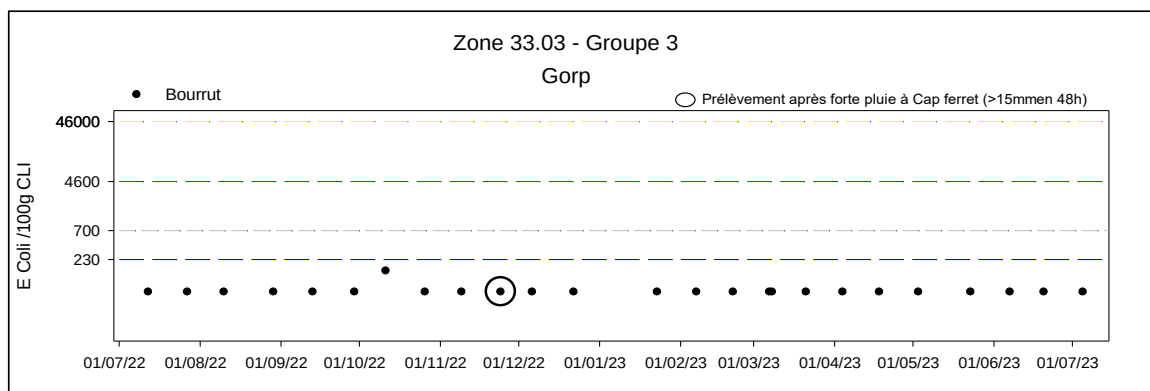
Figure 50: Résultats des analyses en E. coli au point 088-P-019 « Bourrut ».
