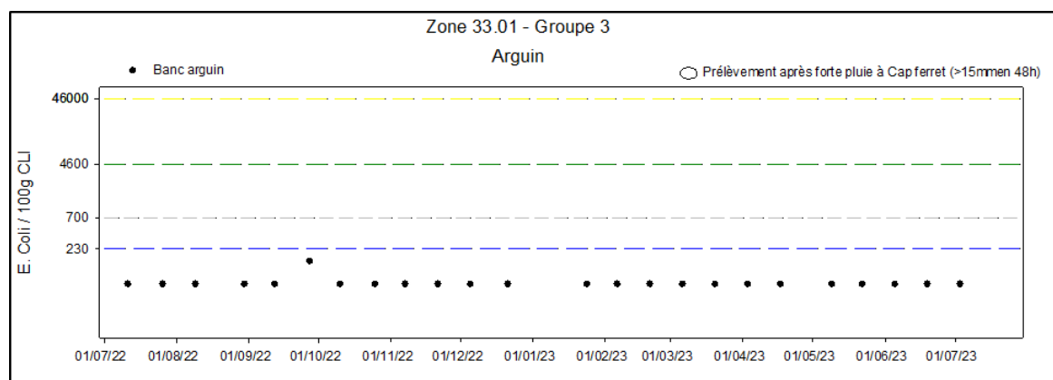
Figure 47 : Résultats des analyses en E. coli au point 087-P-009 « Banc Arguin Sud ».
