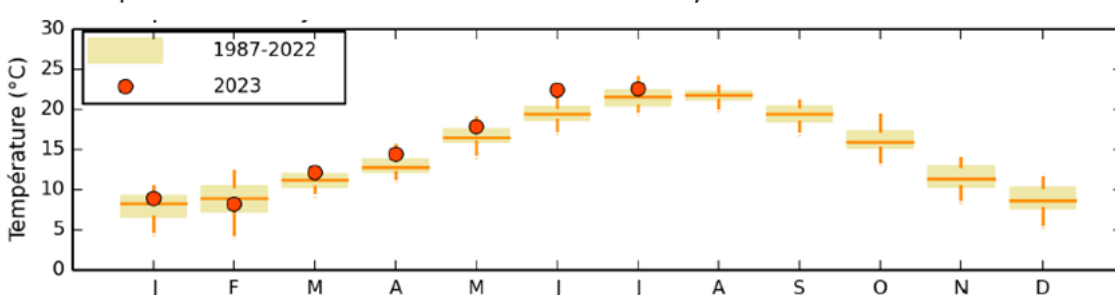
Figure 7 : Synthèse pour les températures de l'air : (a.) moyennes annuelles, (b.) boîtes à moustaches des températures moyennes mensuelles – période 1987-2021 et année 2022, (c.) boîtes à moustaches des températures moyennes mensuelles – période 1987-2022 et année 2023 (source des données Météo France - station de Cap Ferret)
