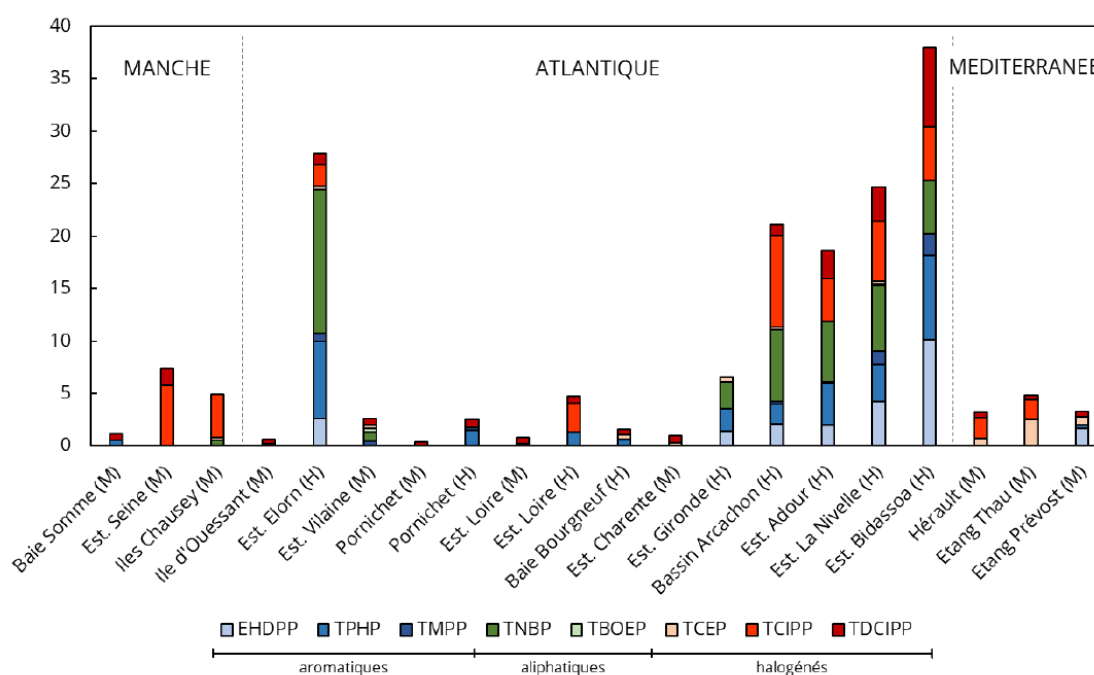
Figure 39 : Concentrations en esters organophosphate en ng g -1 poids sec dans les échantillons de mollusques intertidaux du littoral métropolitain prélevés au mois de novembre 2020
