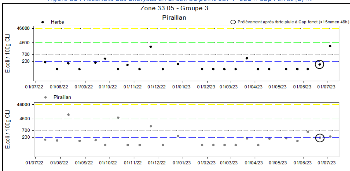
Figure 52 : Résultats des analyses en E. coli aux points «088-P-006 Piraillan » et « 088-P-045 Herbe ».
